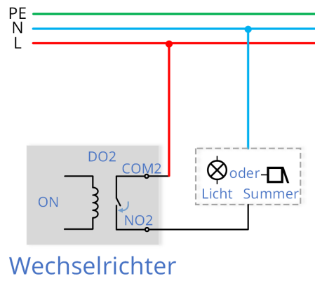
DO2 - Erdschlussalarm
