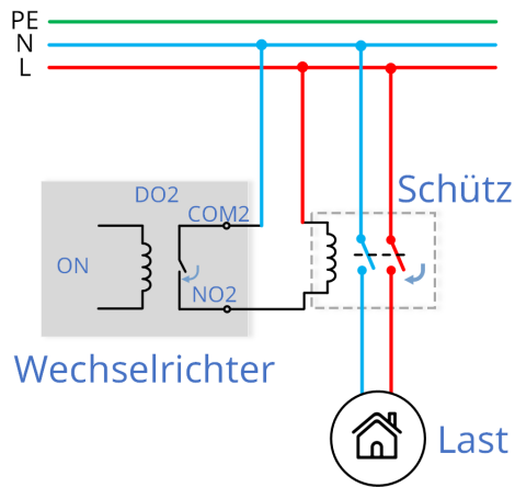
DO2 - Laststeuerung
